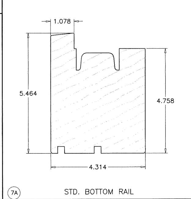
26 HD-PE SILL
